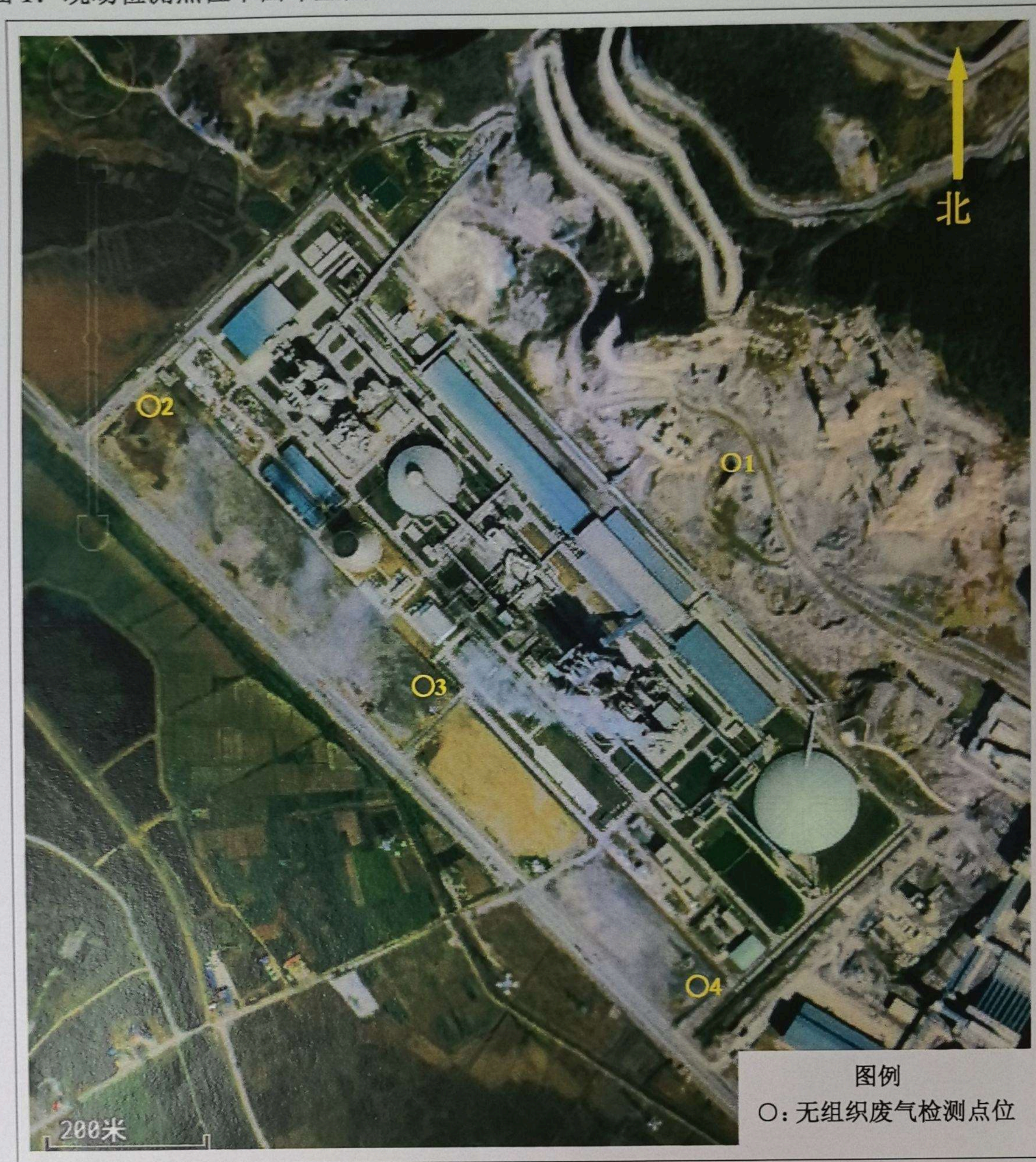
附图 1: 现场检测点位平面布置图
